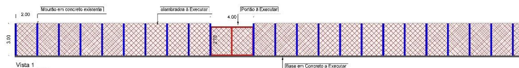
Vista 1 Escala 1:50
