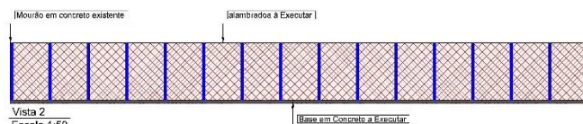
Vista 2 Escala 1:50
